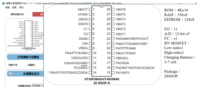
圖 3-22 HT45F8640 28SSOP MCU 選擇簡圖
