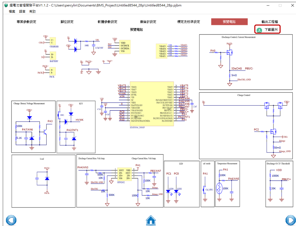
圖 3-43 預覽電路圖
