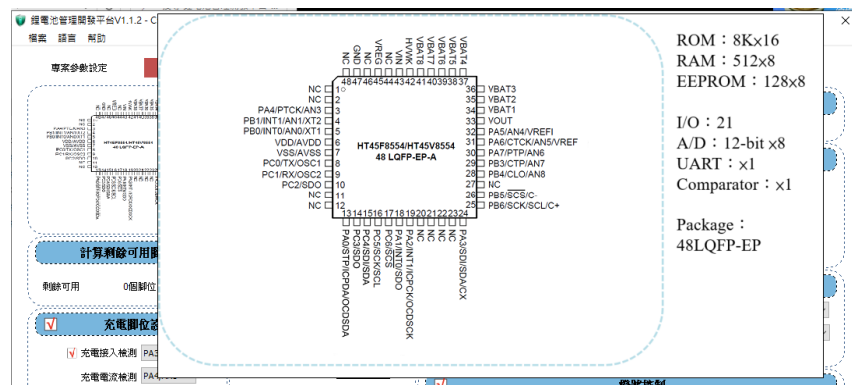
圖 3-20 HT45F8554 48LQFP-EP MCU 選擇簡圖
