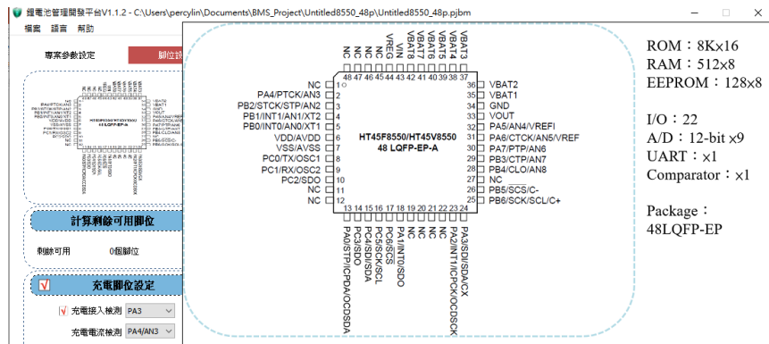
圖 3-16 HT45F8550 48LQFP-EP MCU 選擇簡圖
