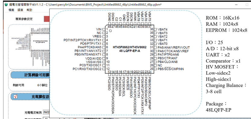
圖 3-25 HT45F8662 48LQFP-EP MCU 選擇簡圖
