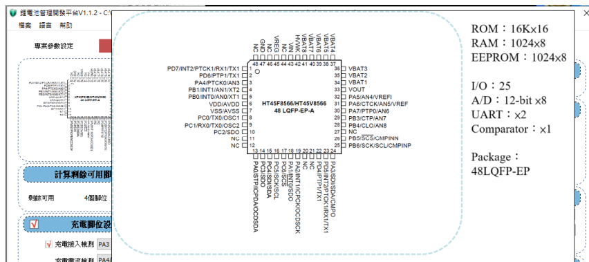
圖 3-21 HT45F8566 48LQFP-EP MCU 選擇簡圖
