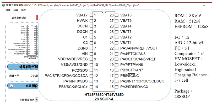
圖 3-23 HT45F8650 28SSOP MCU 選擇簡圖
