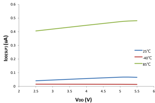
I_{DD(SLP)} VS. V_{DD}
