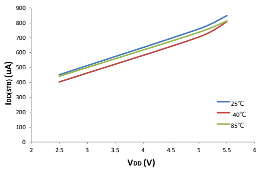
I_{DD(STB)} VS. V_{DD}
