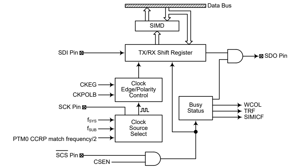
SPI 方框图
