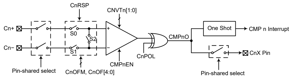
比较器 (n=1)
