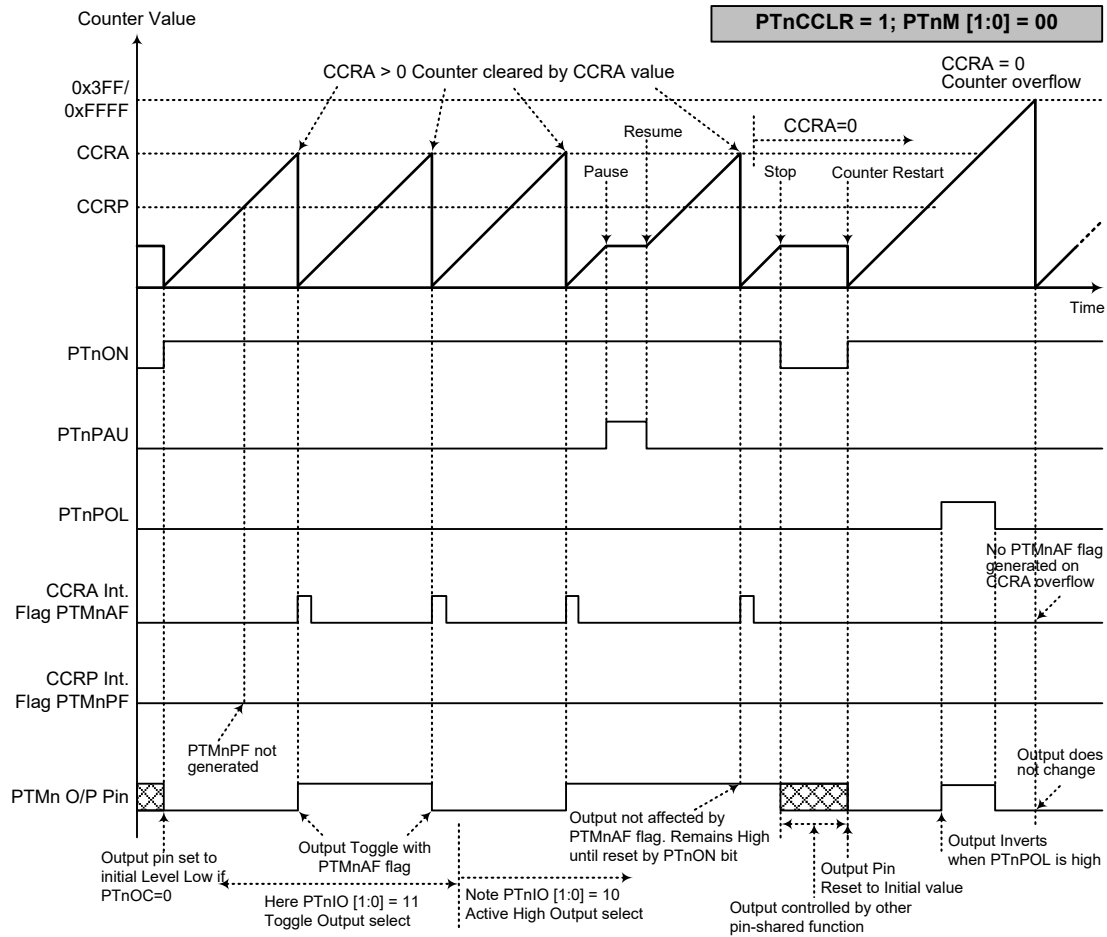
比较匹配输出模式 – PTnCCR=1
