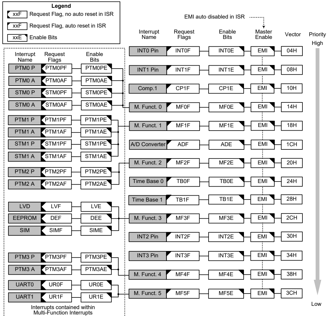
中断结构
