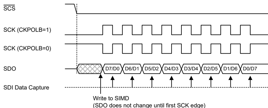
SCK 从机模式时序 - CKEG=0
