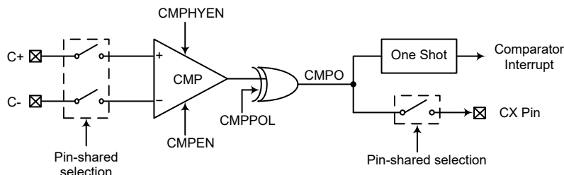
比较器
