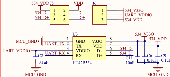
Mini_USB
