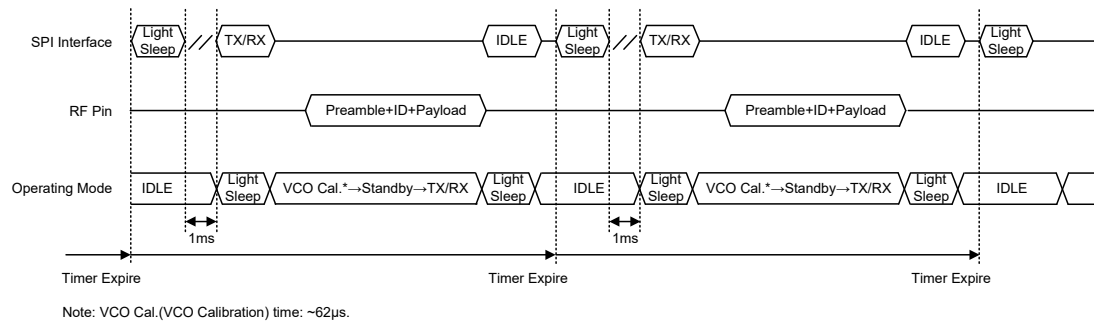
周期性 TX/RX 时序
