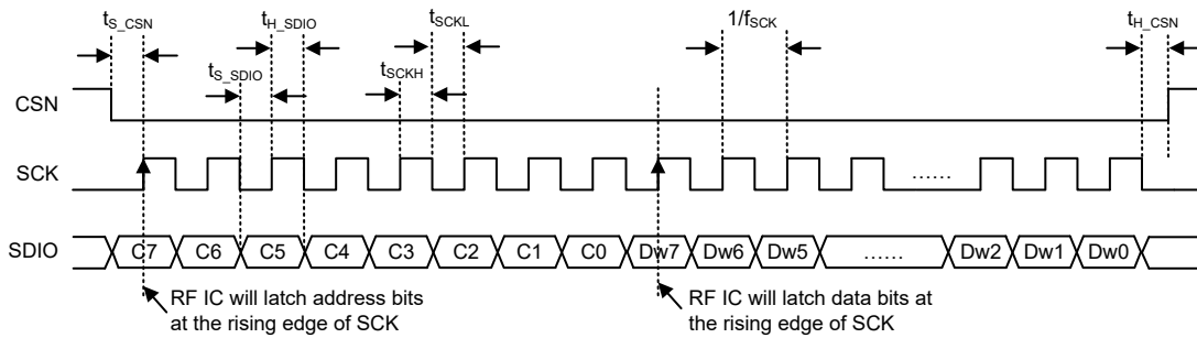
3 线 SPI 接口写入 1 个字节数据
