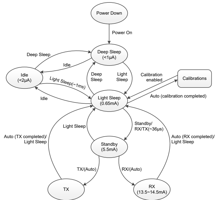
FIFO 模式状态方框图
