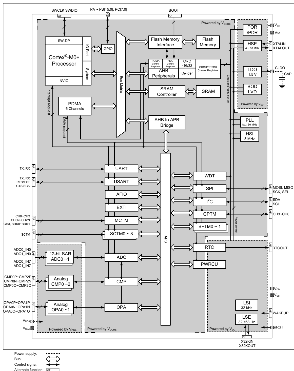
图 1. 方框图
