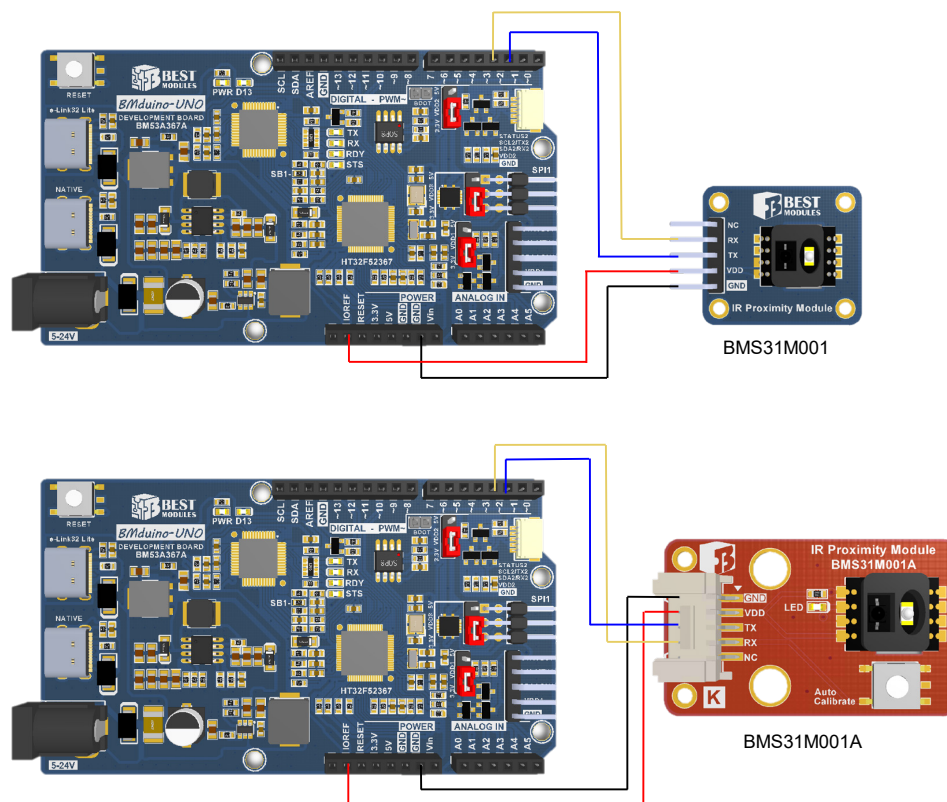
實物連接示意圖
